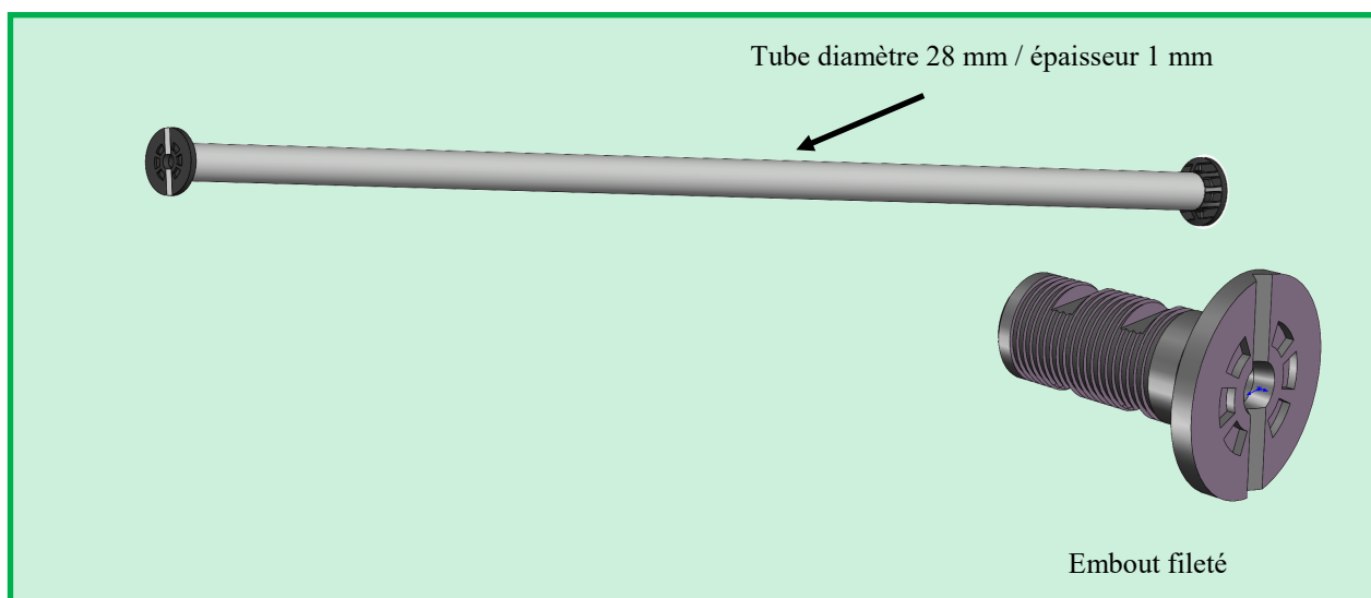
Liernage simple
