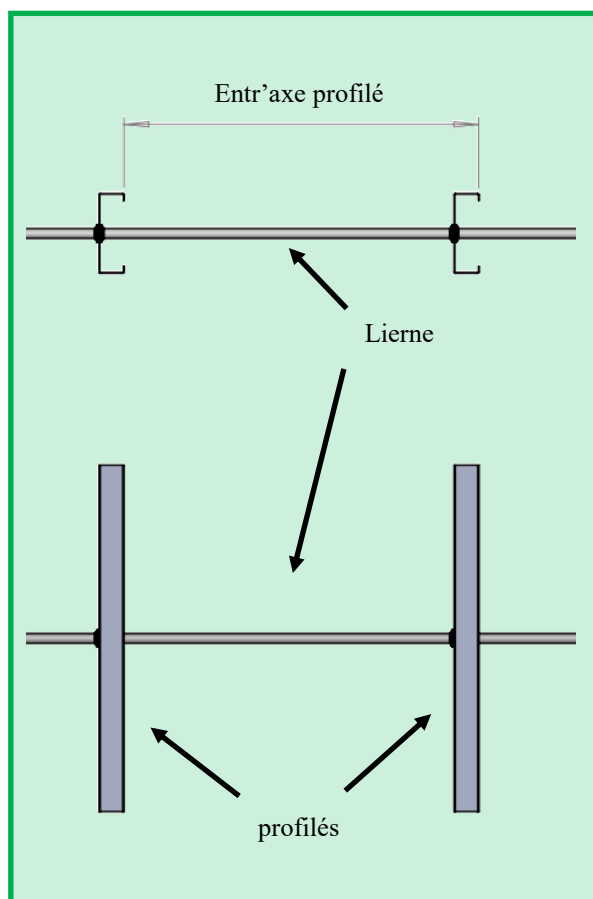
Liernage simple
