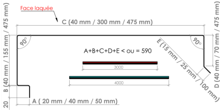
► Coiffe d'acrotère Modèle 8 - Dev 610 mm ◀
