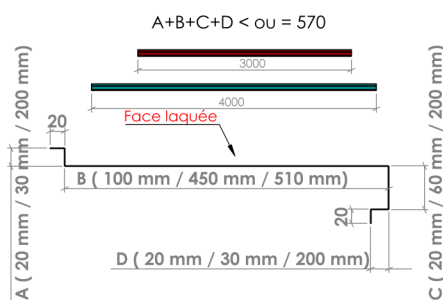
► Rive en solin Modèle 28 - Dev 610 mm ◀
