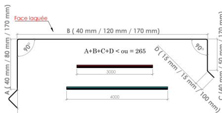
► Coiffe d'acrotère Modèle 7 - Dev 305 mm ◀
