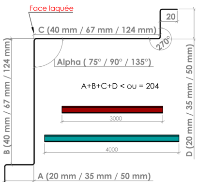
► Raccord d'angle intérieur Modèle 3 - Dev 244 mm ◀
