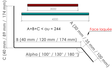
► Rive en solin Modèle 9 - Dev 244 mm ◀
