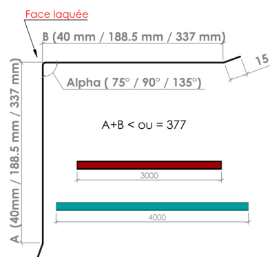
► Raccord d'angle intérieur Modèle 4 - Dev 407 mm ◀
