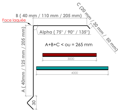
► Rive de pignon Modèle 12 - Dev 305 mm ◀
