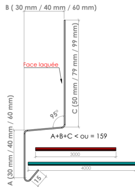
► Larmier ou bavette Modèle 5 - Dev 174 mm ◀
