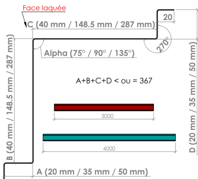
► Raccord d'angle intérieur Modèle 3 - Dev 407 mm ◀
