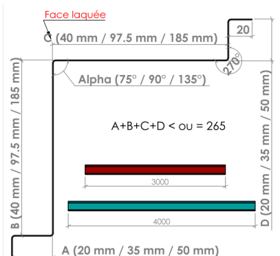
► Raccord d'angle intérieur Modèle 3 - Dev 305 mm ◀
