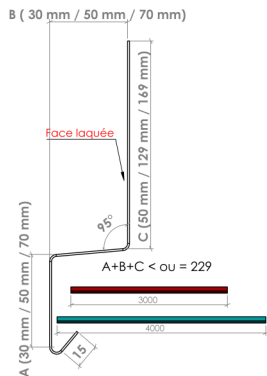
► Larmier ou bavette Modèle 5 - Dev 244 mm ◀
