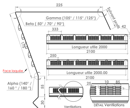
► Faitière simple aérée Modèle 14 - Dev 535 mm ◀
