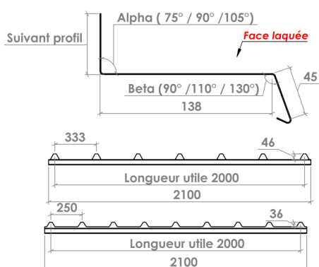
► Cloisoir échancré Modèle 13 - Dev 244 mm ◀
