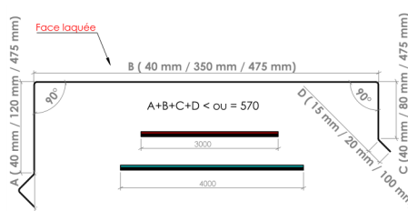
► Coiffe d'acrotère Modèle 7 - Dev 610 mm ◀
