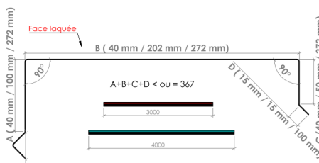
► Coiffe d'acrotère Modèle 7 - Dev 407 mm ◀
