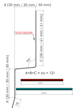
► Larmier ou bavette Modèle 6 - Dev 136 mm ◀
