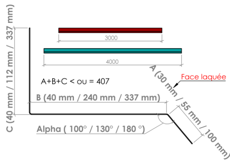
► Rive en solin Modèle 9 - Dev 407 mm ◀
