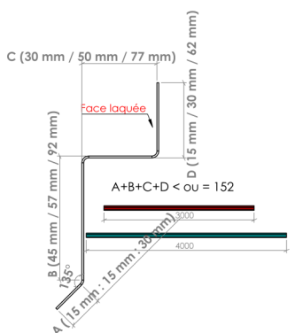
► Rive en solin Modèle 11 - Dev 152 mm ◀
