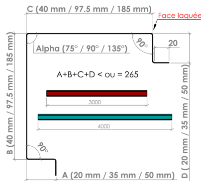
► Raccord d'angle extérieur Modèle 1 - Dev 305 mm ◀
