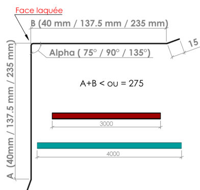
► Raccord d'angle intérieur Modèle 4 - Dev 305 mm ◀
