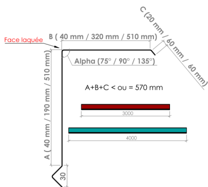
► Rive en solin Modèle 12 - Dev 610 mm ◀
