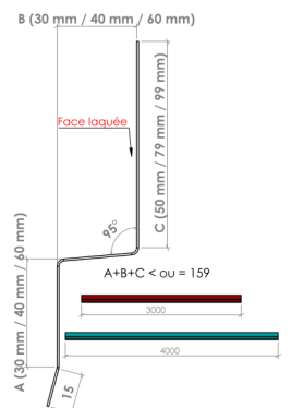
► Larmier ou bavette Modèle 6 - Dev 174 mm ◀
