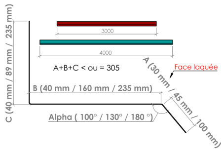
► Rive en solin Modèle 9 - Dev 305 mm ◀
