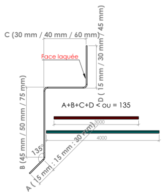
► Rive en solin Modèle 11 - Dev 135 mm ◀
