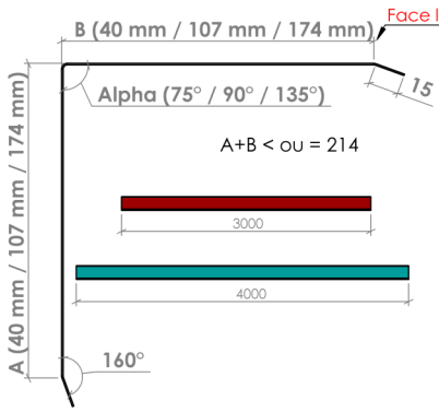
► Raccord d'angle extérieur Modèle 2 - Dev 244 mm ◀
