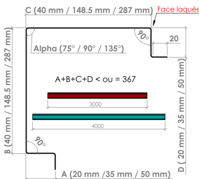
► Raccord d'angle extérieur Modèle 1 - Dev 407 mm ◀
