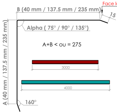
► Raccord d'angle extérieur Modèle 2 - Dev 305 mm ◀
