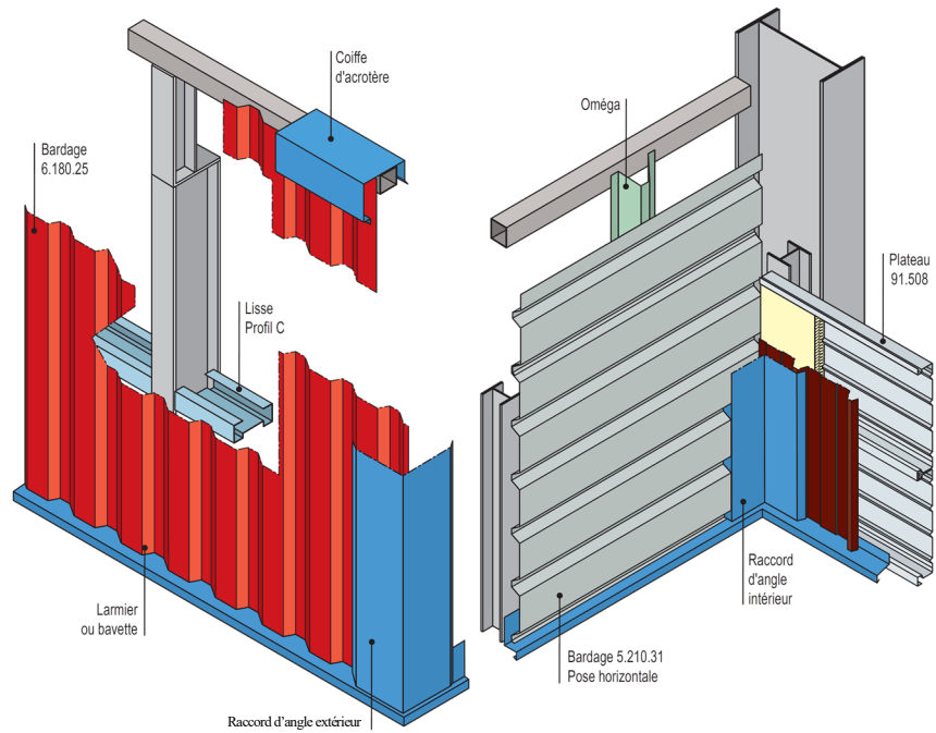
► Raccord d'angle extérieur Modèle 1 - Dev 244 mm ◀
