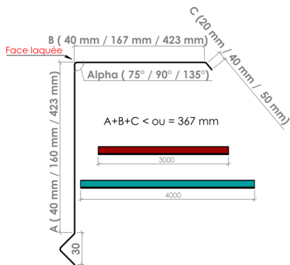
► Rive en solin Modèle 12 - Dev 407 mm ◀
