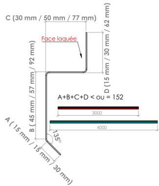
► Rive en solin Modèle 10 - Dev 152 mm ◀
