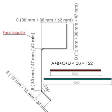
► Rive en solin Modèle 10 - Dev 122 mm ◀
