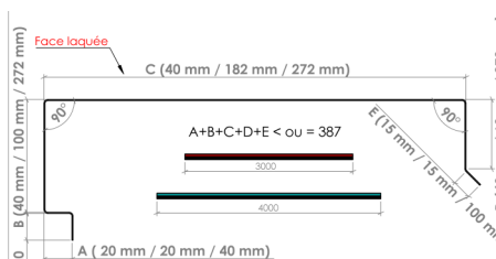
► Coiffe d'acrotère Modèle 8 - Dev 407 mm ◀
