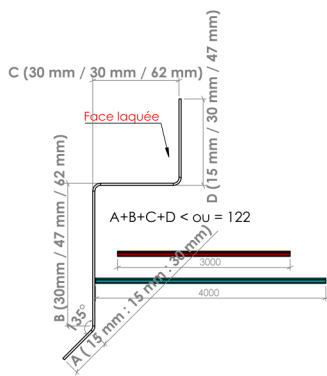
► Rive en solin Modèle 11 - Dev 122 mm ◀
