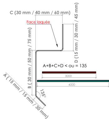
► Rive en solin Modèle 10 - Dev 135 mm ◀
