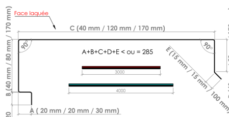
► Coiffe d'acrotère Modèle 8 - Dev 305 mm ◀
