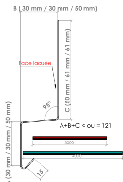
► Larmier ou bavette Modèle 5 - Dev 136 mm ◀
