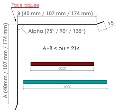
► Raccord d'angle intérieur Modèle 4 - Dev 244 mm ◀
