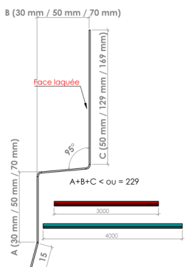
► Larmier ou bavette Modèle 6 - Dev 244 mm ◀
