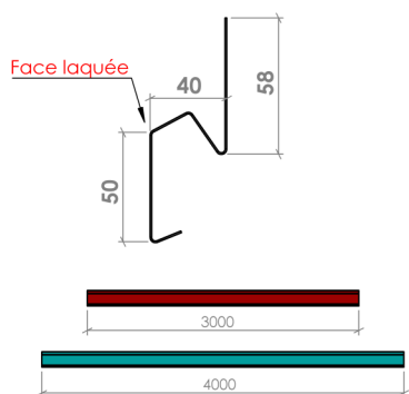
► lame de départ Modèle 26 - Dev 174 mm ◀
