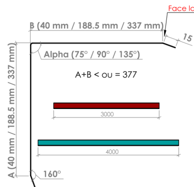
► Raccord d'angle extérieur Modèle 2 - Dev 407 mm ◀
