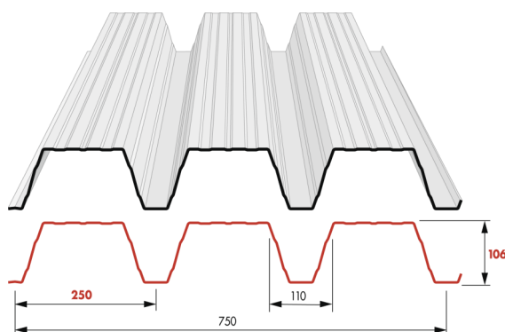
CARACTÉRISTIQUES GÉOMÉTRIQUES
