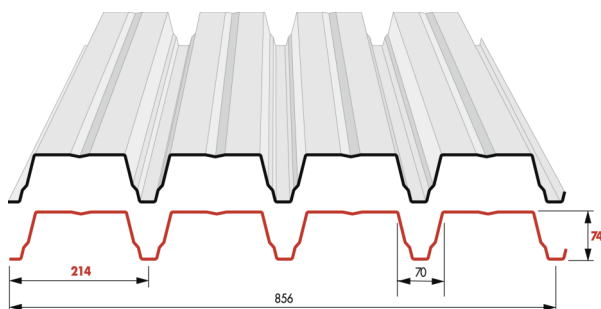
CARACTÉRISTIQUES GÉOMÉTRIQUES
